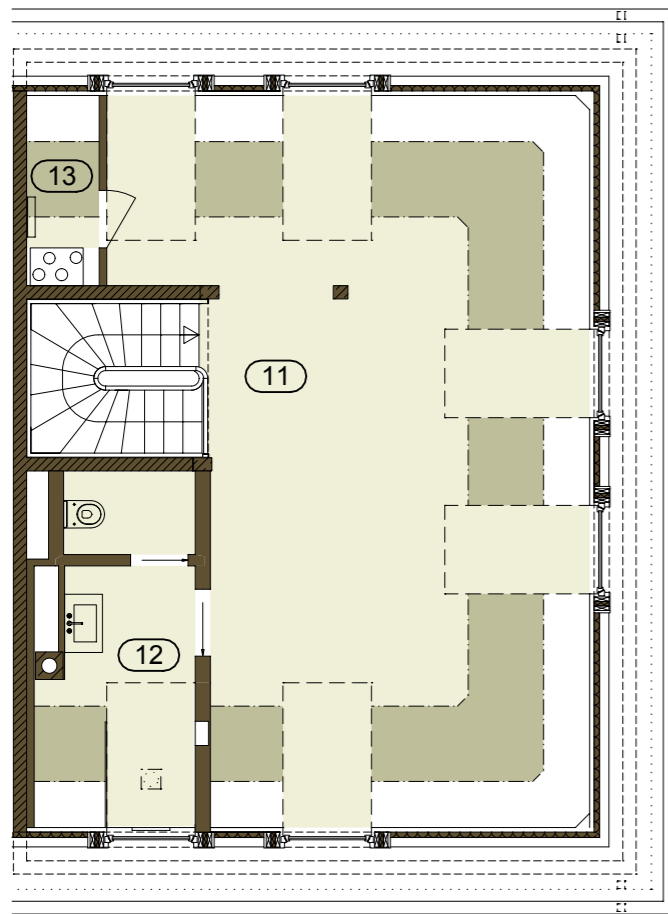
DACHGESCHOSS
