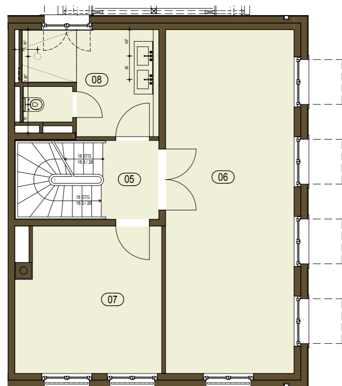
OBERGESCHOSS
