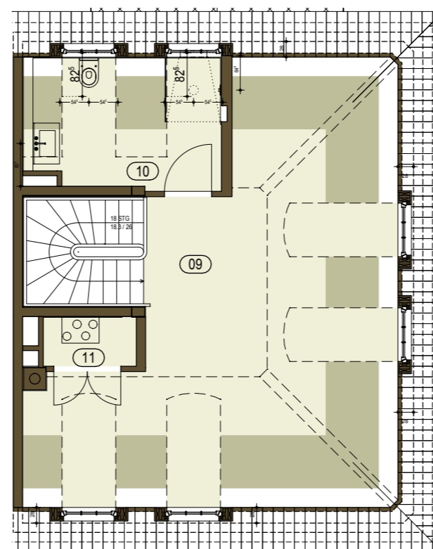
DACHGESCHOSS
